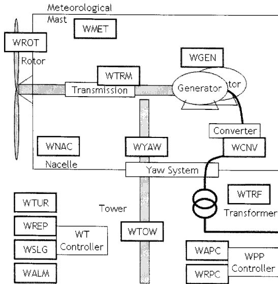
그림 2 풍력발전시스템의 LN 구성 Fig. 2 LN Configuration of Wind Power Generation System
