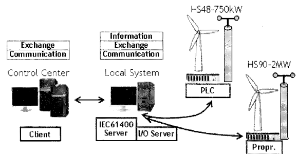
그림 3 통신 Interface 구성도 Fig. 3 Configuration of Communication Interface
