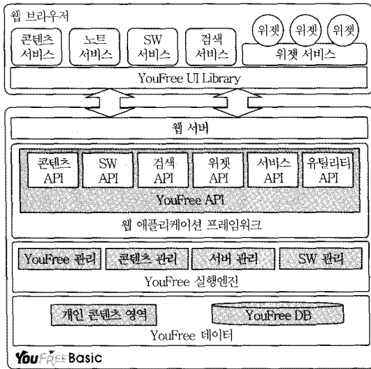
(그림 2) 개인용 소프트웨어 플랫폼-YouFree Basic의 구조
