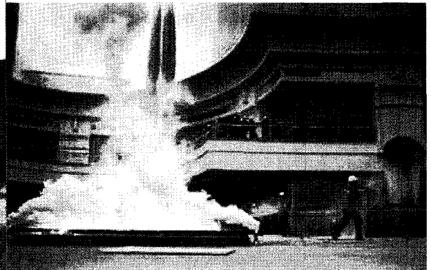
<사진 5> 실제크기 화재시험 장면
