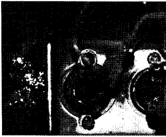
〈그림7〉 연소되었으나 정상인 서모스탯 전극
