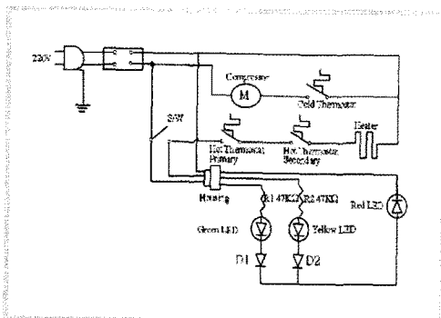
〈그림2〉 냉온수기의 회로도 한 예
