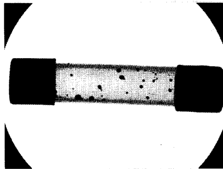
〈그림11〉 전원퓨즈의 내부 비산 흔적(과전류)
