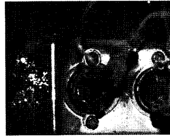
〈그림9〉 내부배선의 금속부에 의한 절연파괴
