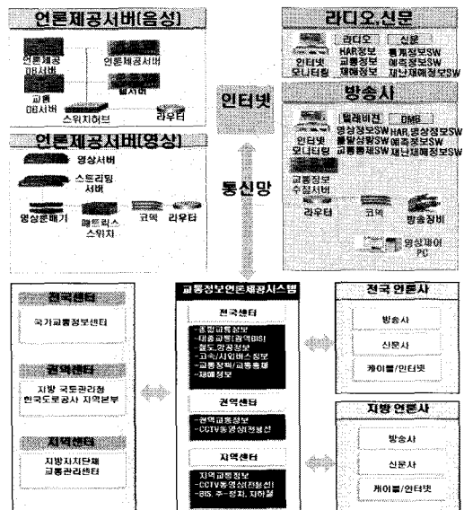
그림 11. 교통정보 언론제공 연계시스템 Fig. 11. Traffic information press system 교통정보 언론제공 연계시스템의 언론기관 운영 단말기는
