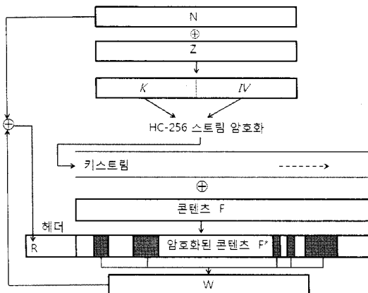
그림 3. 플레이어 카피 \langle id, pw, Z, L \rangle 를 위해 서버에서 콘텐츠 파일 F 를 암호화 하는 과정
