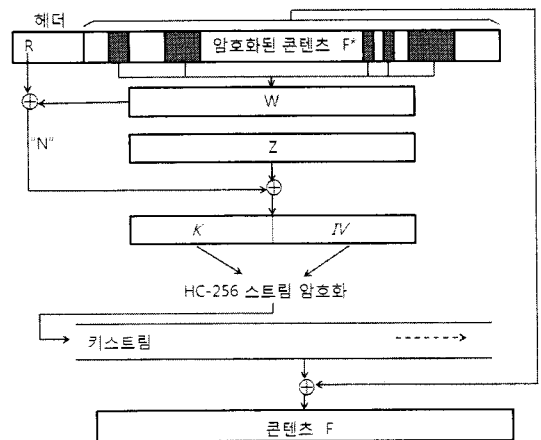
그림 4. 플레이어 카피 \langle id, pw, Z, L \rangle 에서 암호화된 콘텐츠 F^* 를 복호화 하는 과정
