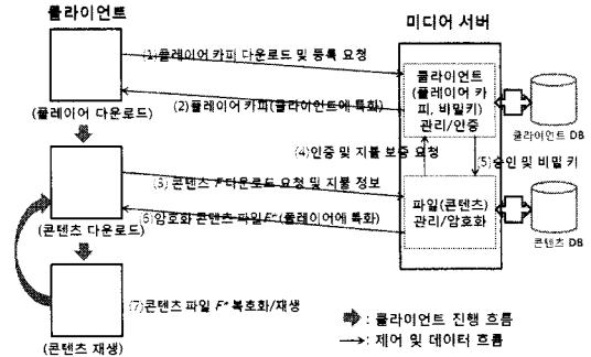
그림 1. 제안 구조상의 클라이언트-서버 상호 작용
