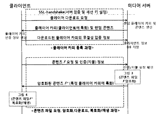
그림 2. 클라이언트-서버 사이의 전체 과정 흐름도
