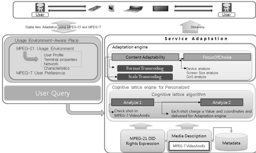
(그림 1) UP-SAM 모델 구조
