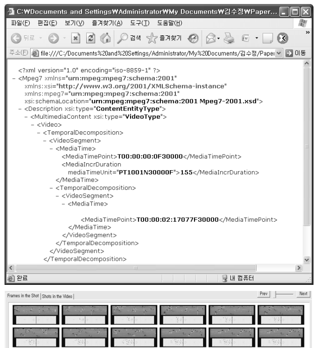
(그림 2) 프레임을 샷으로 나누는 과정
