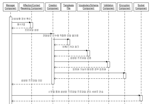
(그림 4) 사용자 단말기 플랫폼 시작시 프로파일 관리서버와의 시퀀스 다이어그램
