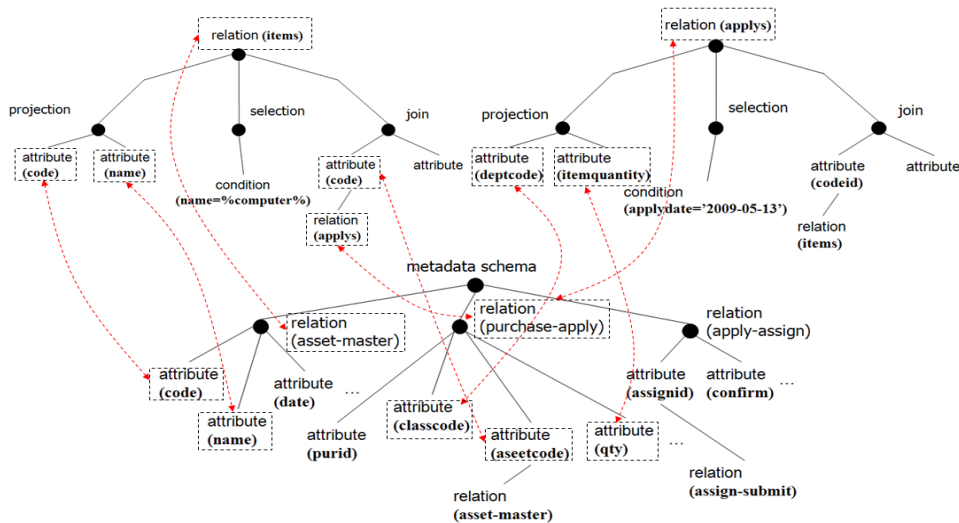
(그림 11) 글로벌 쿼리와 로컬 쿼리 매핑 과정
