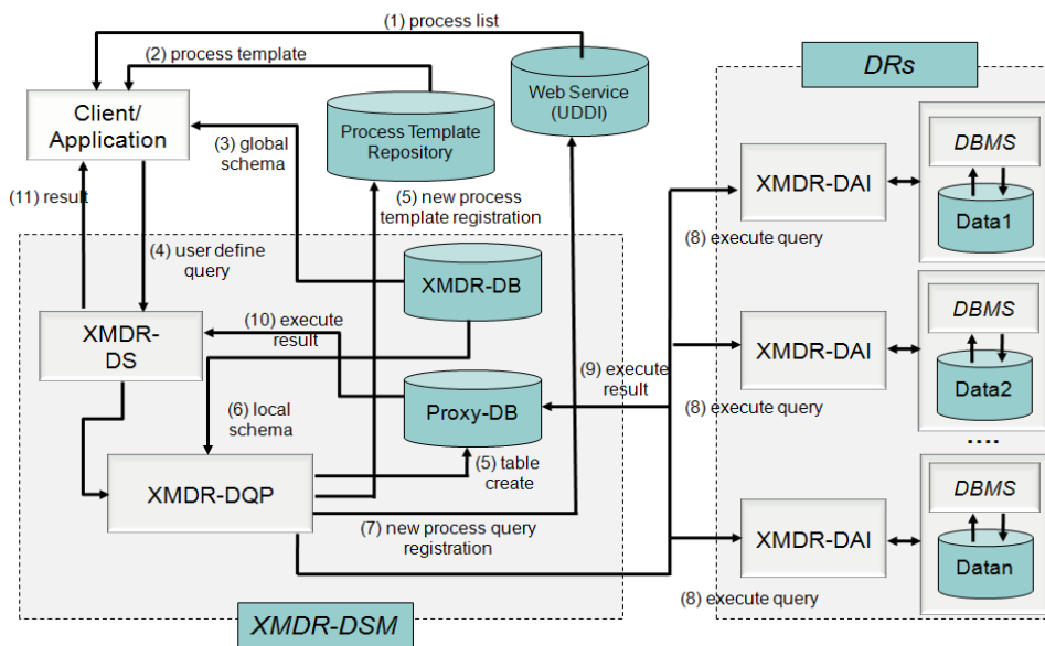
(그림 3) 협업 시스템 전체 흐름
