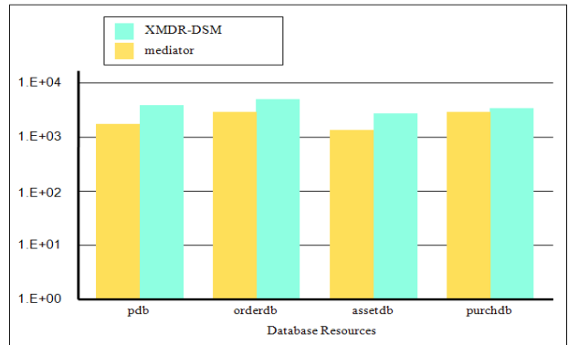
(그림 21) 쿼리 수행 처리 시간 비교
