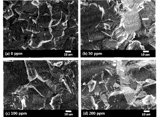
그림 5. 1700°C에서 5시간 소결한 보호막의 Fe 2 O 3 첨가량 변화(x =0, 50, 100, 200)에 따른 파단면의 SEM 사진.
