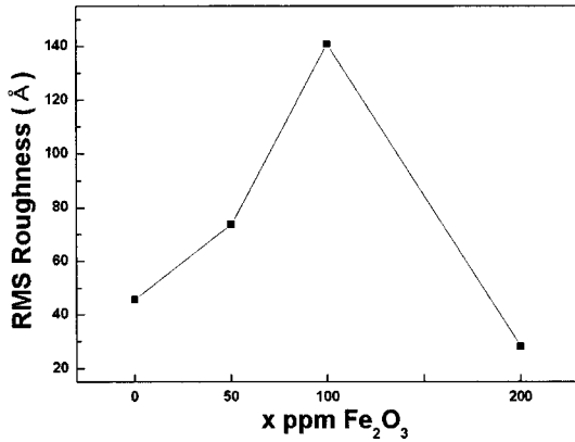
그림 9. 첨가량 변화에 따른 MgO 박막의 표면거칠기.
