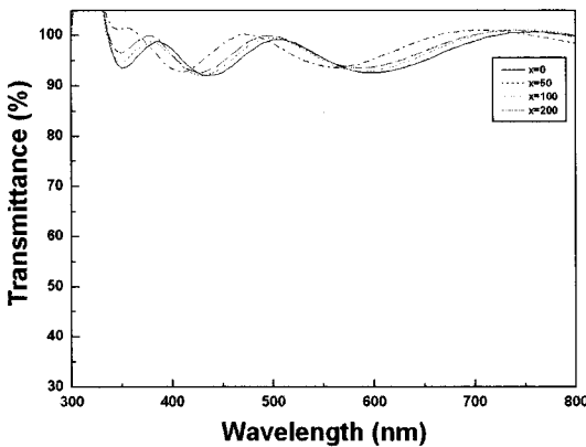
그림 10. 첨가량 변화에 따른 MgO 박막의 가시광영역에서의 투과율.
