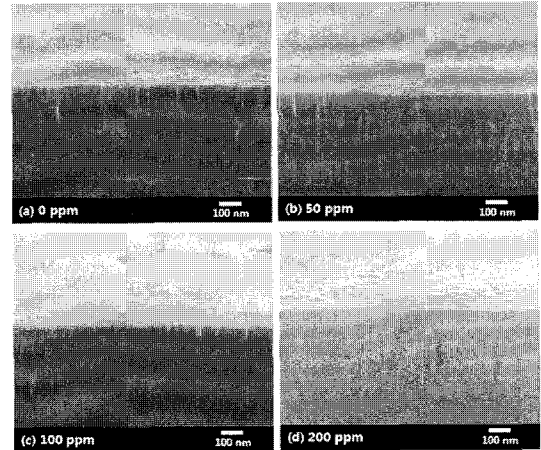
그림 7. Fe 2 O 3 첨가량에 따른 MgO 박막의 FE-SEM 사진. Fig. 7. FE-SEM images of MgO + x ppm Fe 2 O 3 films as a function of Fe 2 O 3 content. (a) x=0 , (b) x=50 , (c) x=100 , (d) x=200
