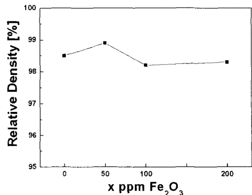
그림 2. Fe 2 O 3 첨가량에 따른 상대밀도. Fig. 2. Relative density of MgO + x ppm Fe 2 O 3 as a function of Fe 2 O 3 content.
