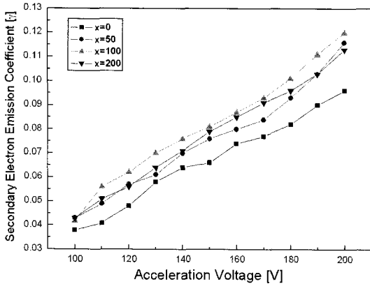
그림 6. 첨가량 변화에 따른 2차전자방출계수. Fig. 6. The secondary electron emission coefficient of MgO + x Fe 2 O 3 films as a function of Fe 2 O 3 content.
