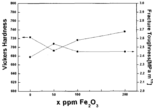
그림 3. 첨가량 변화에 따른 소결체의 비커스 경도값.
