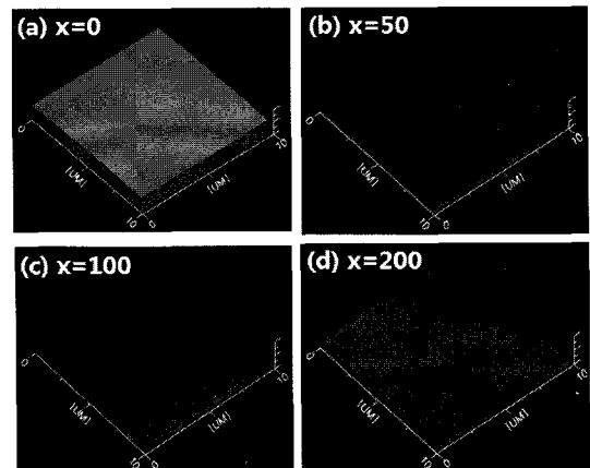
그림 8. Fe 2 O 3 첨가량 변화에 따른 MgO 박막의 AFM사진. Fig. 8. AFM images of MgO + x ppm Fe 2 O 3 films as a function of Fe 2 O 3 content. (a) x=0 , (b) x=50 , (c) x=100 , (d) x=200
