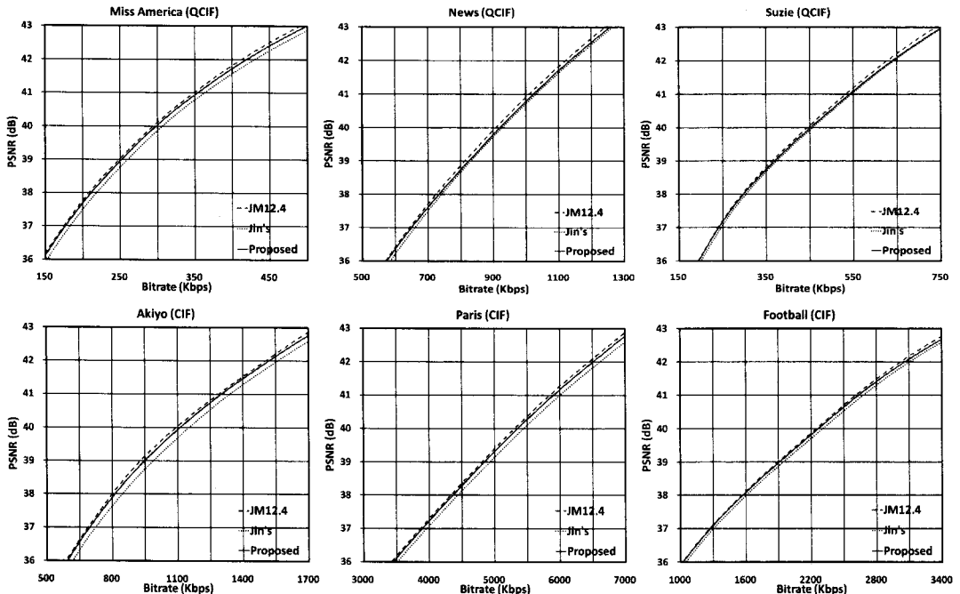
그림 9. 객관적 화질(PSNR)이 36~43 dB를 갖는 영역에서 (a) QCIF 영상(Miss America, News, Suzie) 및 (b) CIF 영상(Akiyo, Paris, Football)에 대한 윌-왜곡 곡선 (rate-distortion curve)
