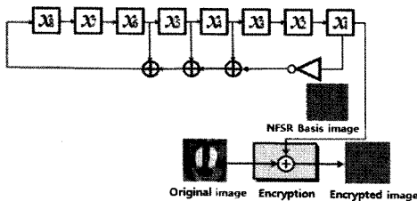
그림 3. 제안된 NFSR 구조 Fig. 3. Proposed NFSR structure
