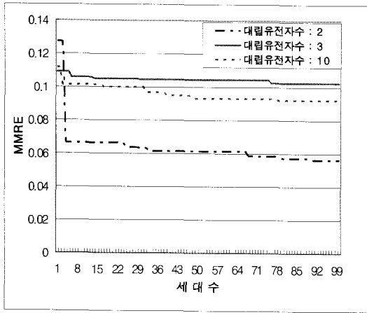
그림 7. 훈련 데이터의 세대수에 따른 MMRE 비교 Fig. 7. MMRE comparison by populations of training set
