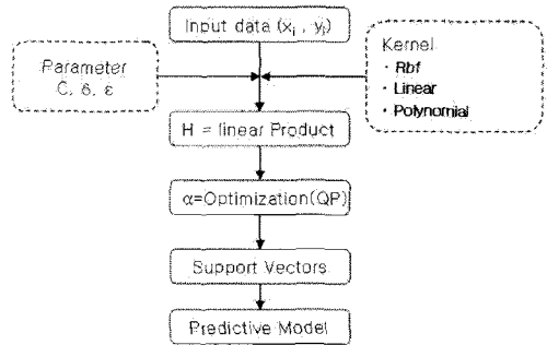
그림 1. SVR 처리 순서도 Fig. 1. Flowchart of SVR
