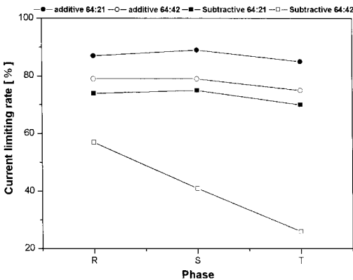
그림 7. R, S, T 상의 전류제한률. Fig. 7. Current limiting rate of R, S, T phase.
