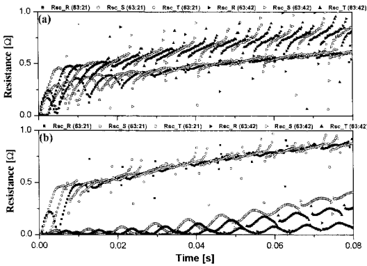
그림 6. 저항 파형 (a:가극 결선, b:감극 결선). Fig. 6. Resistance pattern (a: additive polarity, b: subtractive polarity).
