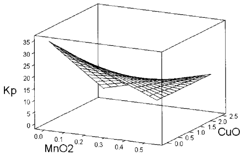
그림 6. 최적소결온도에서 소결한 (\text{Na}_{1/2}\text{K}_{1/2})\text{NbO}_3 조성의 \text{CuO} 및 \text{MnO}_2 첨가량에 따른 전기기계결합계수( K_p ).
