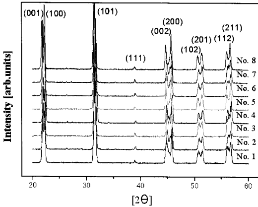
그림 1. 최적 소결온도에서 소결한 (Na 1/2 K 1/2 )NbO 3 조성의 CuO 및 MnO 2 첨가량에 따른 XRD 결과.
