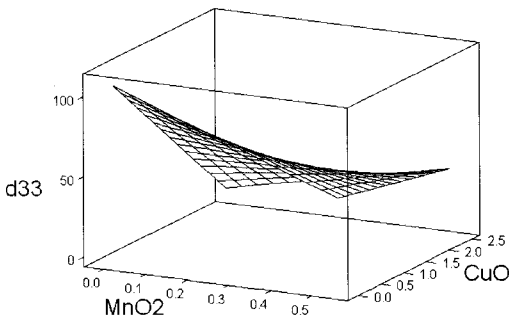
그림 7. 최적소결온도에서 소결한 (\text{Na}_{1/2}\text{K}_{1/2})\text{NbO}_3 조성의 \text{CuO} 및 \text{MnO}_2 첨가량에 따른 압전상수( d_{33} ).
