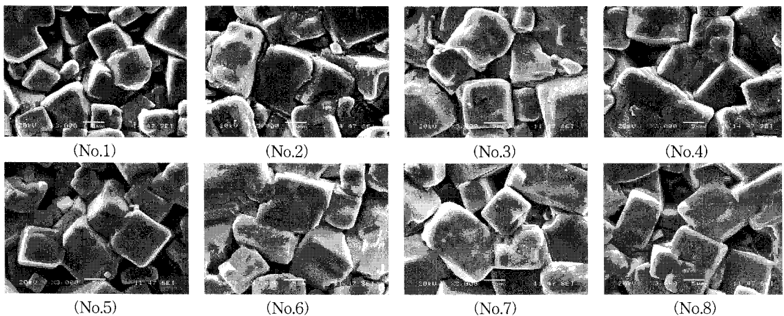
그림 2. 최적 소결온도에서 소결한 (Na 1/2 K 1/2 )NbO 3 조성의 CuO 및 MnO 2 첨가량에 따른 SEM 사진.
