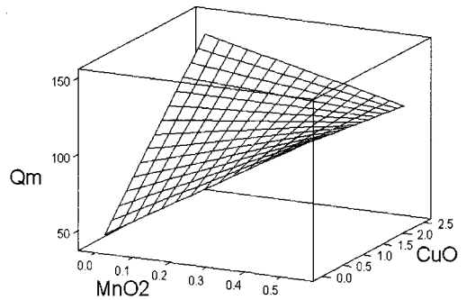
그림 5. 최적소결온도에서 소결한 (\text{Na}_{1/2}\text{K}_{1/2})\text{NbO}_3 조성의 \text{CuO} 및 \text{MnO}_2 첨가량에 따른 기계적 품질계수( Q_m ).
