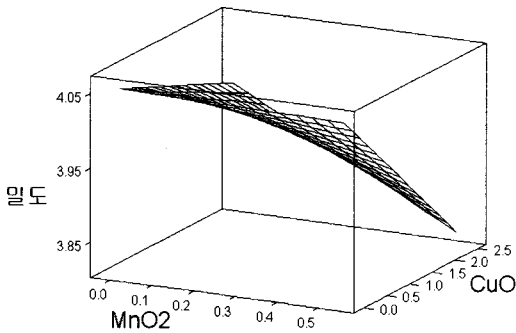
그림 3. 최적 소결온도에서 소결한 (\text{Na}_{1/2}\text{K}_{1/2})\text{NbO}_3 조성의 \text{CuO} , \text{MnO}_2 첨가량에 따른 밀도.
