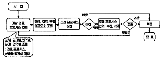
그림 3. 소프트웨어 개발 경로 프로세스 조정 흐름도 Fig 3. Software development path and process chart
