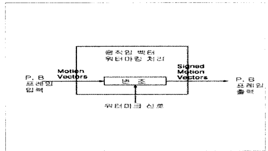
그림 2. P, B 프레임의 워터마킹 과정 Fig 2. Watermarking process of P, B frame
