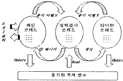
[그림 2] 순음청력검사 시스템의 쓰레드 모델
