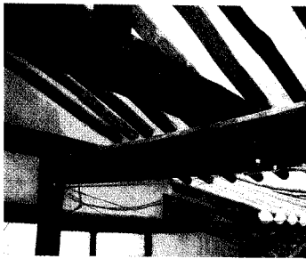
안대청 가구구조
