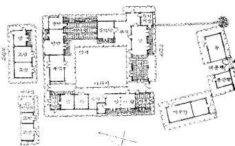
두곡고택 (도면출처 : 한국정신문화연구원)
