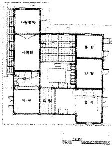
본체 평면도(도면출처 : 김화봉)
