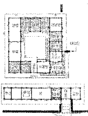
서백당 (도면출처 : 강영환)
