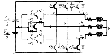
Mode vi; v_{an}=V_{dc}; v_{bn}=\frac{V_{dc}}{2}, v_{cn}=0
