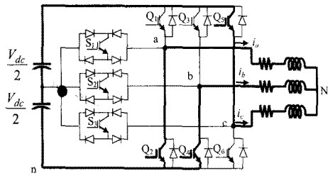
Mode i; v_{an}=0; v_{bn}=0, v_{cn}=V_{dc}
