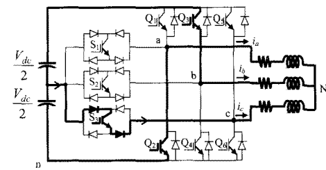
Mode x; v_{an}=0; v_{bn}=V_{dc}, v_{cn}=\frac{V_{dc}}{2}
