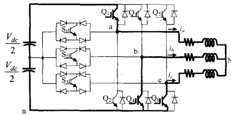
Mode v; v_{an}=V_{dc}; v_{bn}=0, v_{cn}=0
