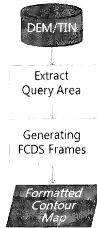
그림 3. FCM 생성 단계 Fig. 3 FCM Generation Steps
