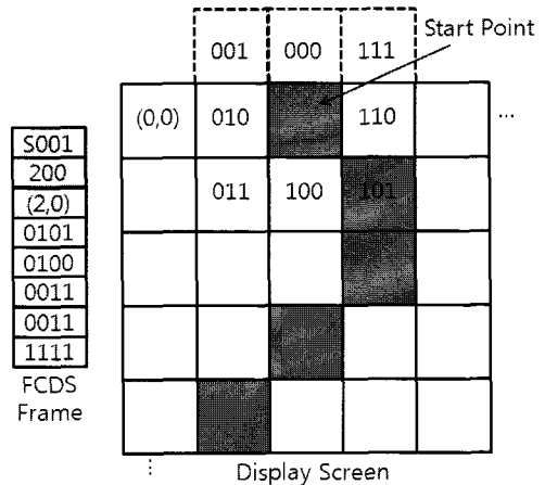
그림 2. FCDS와 Client 출력 Example Fig. 2 Example of FCDS and Client Display
