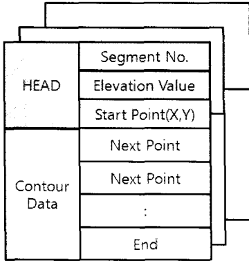
그림 1. FCDS 프레임 형식 Fig. 1 FCDS Frame Format
