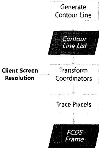
그림 4. FCDS 생성 단계 Fig. 4 FCDS Generation Steps
