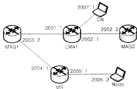
그림 3-2. 시험 네트워크
