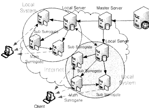
그림 1. 제안한 RDCDN의 구조 Figure 1. The Proposed Architecture of RDCDN Model
