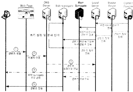
그림 5. 클라이언트까지의 전송 과정 Figure 5. The Procedure of Delivering Contents to RDCDN Clients
