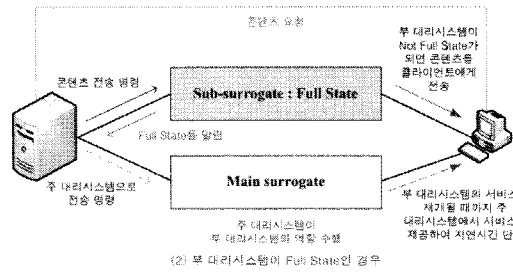
그림 4. 전송 알고리즘의 효율성 Figure 4. The Efficiency of RDCDN Transmission Algorithm
