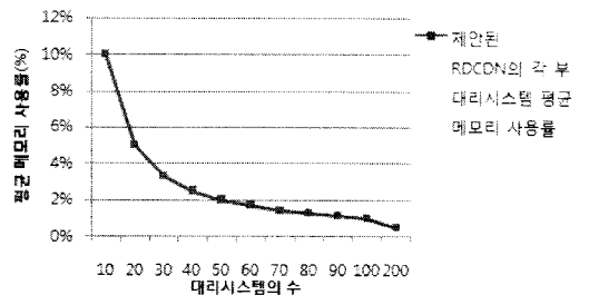
그림 6. RDCDN 부 대리시스템의 메모리 사용률 Figure 6. Average Storage Space Occupation Rate of Sub-Surrogate of RDCDN
