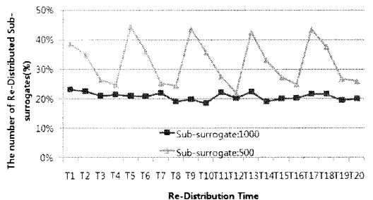
그림 8. 부 대리시스템 개수에 따른 재분배에 참여하는 부 대리시스템의 비율 비교 Figure 8. Comparison of Re-distribution Rate (Sub-surrogates)
