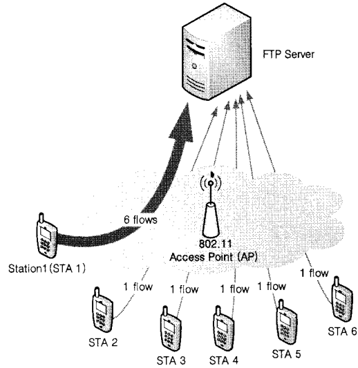
그림 1. 다수의 TCP 업링크 스트림을 갖는 STA에 의한 전송대역폭 독점 현상 재연을 위한 시뮬레이션 환경
