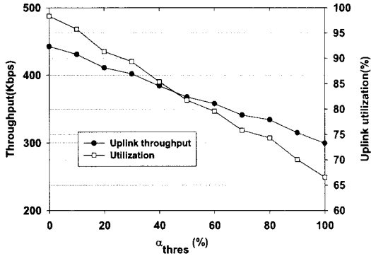
그림 6. \alpha_{thres} 값 설정에 따른 업링크 throughput과 utilization
