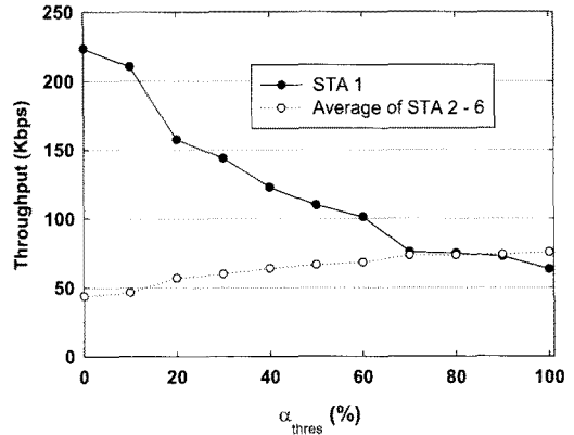
그림 5. \alpha_{thres} 값 설정에 따른 STA별 throughput 변환
