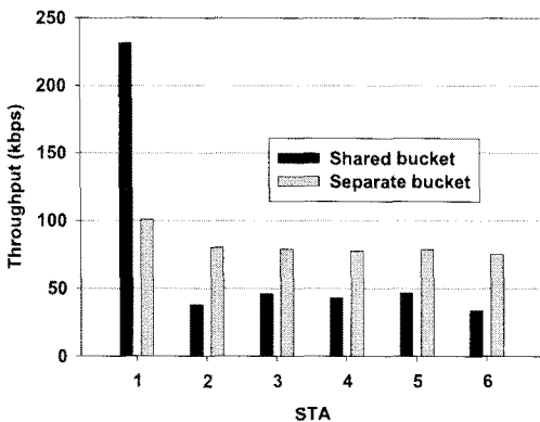
그림 4. TCP 업링크의 STA별 throughput
