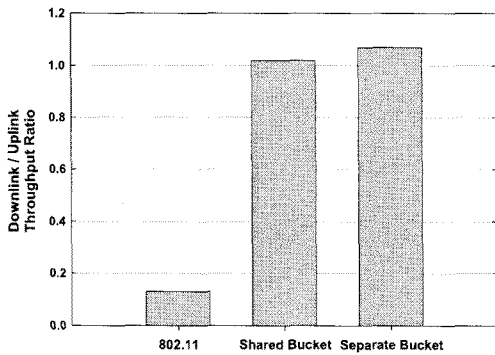
그림 3. TCP 업링크와 다운링크 throughput 간 비율
