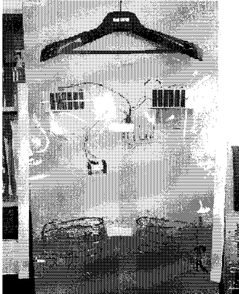
[그림 4] 솔라셀을 이용한 히터 재킷
