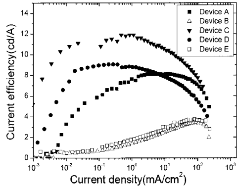
그림 3. 청색 인광 OLEDs의 전류효율-전류밀도 곡선.
