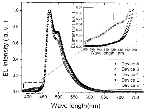
그림 4. 청색 인광 OLEDs의 EL 스펙트럼. Inset : 380-450 nm 구간의 확대 스펙트럼.
