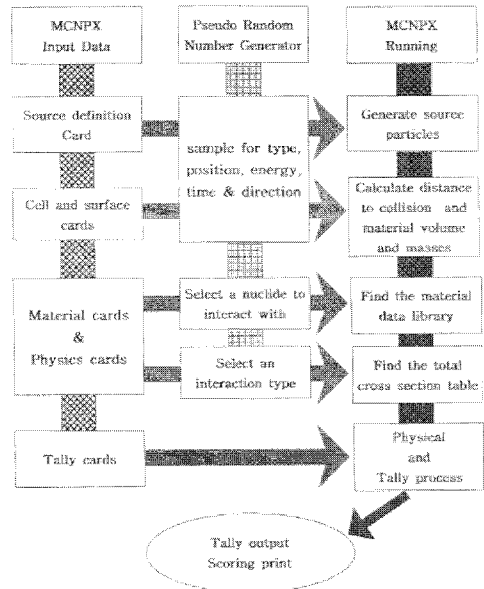
그림 1. MCNP 코드 계산 알고리즘[10].
