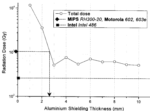
그림 5. 10년간 반도체에 흡수되는 총 선량.
