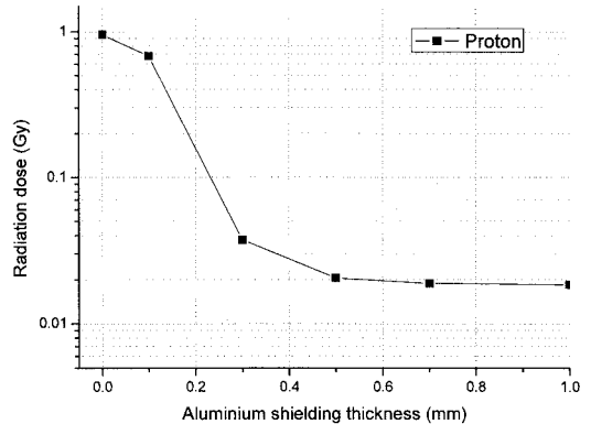
그림 4. 세부 양성자 흡수선량 계산. Fig. 4. Detailed proton radiation dose calculation.
