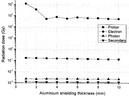
그림 3. 알루미늄 두께에 따른 흡수선량. Fig. 3. Radiation dose of the semiconductor as the aluminium thickness.
