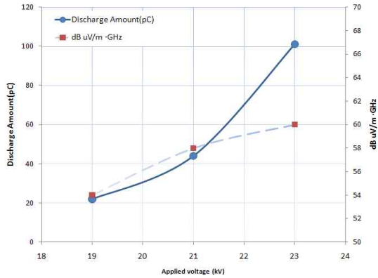
그림 3. 전압인가별 결보기방전량과 전자기파 방전신호의 크기.
