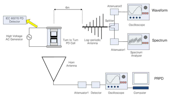
그림 2. 부분방전에 의한 방사 전자기파 측정 실험구성.
