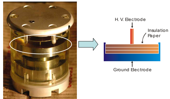
그림 1. 금속이물 방전을 모의한 PD cell.
