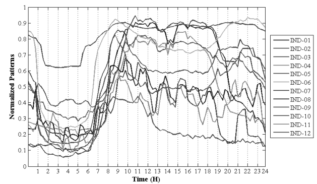
(그림 9) 산업용 대표 프로파일
