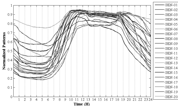
(그림 7) 일반용 대표 프로파일
