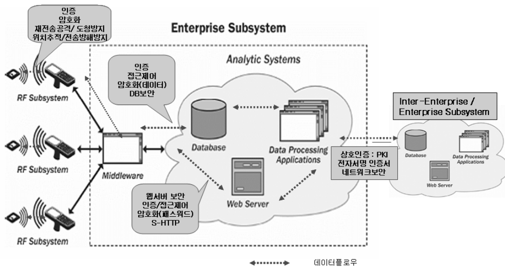
(그림 2) RFID Enterprise Subsystem
