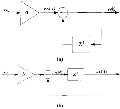
그림 6. I와 Q 채널의 루프 필터 구조 (a) I 채널 (b) Q 채널 Fig. 6. Loop filter structure of I and Q channel. (a) I channel (b) Q channel
