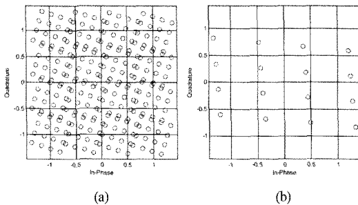
그림 3. IQ 불균형에 의해 왜곡된 신호의 성상도 (16 QAM). (a) 다중 반송파 시스템 (b) 단일 반송파 시스템 Fig. 3. Constellation point of distorted signal due to the IQ imbalance (16 QAM). (a) Multi-carrier system (b) Single-carrier system
