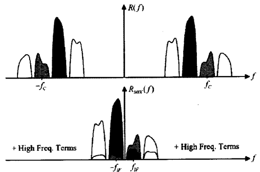
그림 2. 수신된 신호 r(t) 와 mixer 를 통해 출력된 rMIX(t) 의 스펙트럼. Fig. 2. Spectra of the received signal r(t) and the mixer output signal rMIX(t) .
