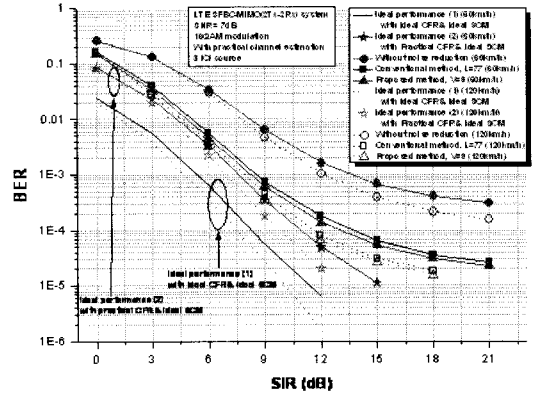
(b) LTE SFBC-MIMO 시스템
