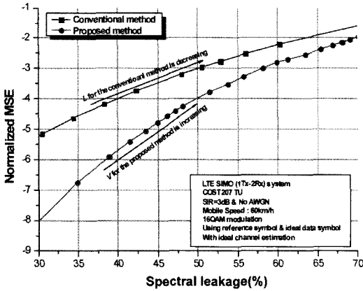
그림 4. Spectral leakage에 따른 기존의 방식과 제안된 방식의 추정된 covarianc에 대한 normalized MSE 성능 비교
