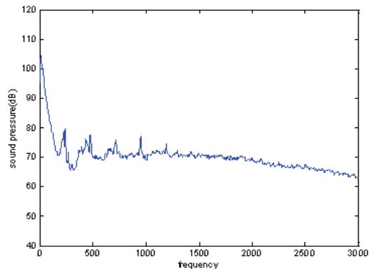
Fig. 1 Fan noise spectrum
