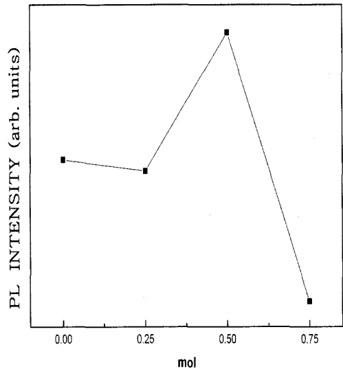
그림 5. x 의 다양한 변화에 따른 (Zn_{1-x}Mg_x)_2SiO_4:Mn 발광스펙트럼 변화.
