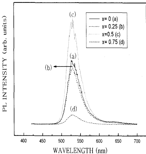
그림 4. x 의 변화에 따른 (Zn_{1-x}Mg_x)_2SiO_4:Mn 광 여기 발광스펙트럼.
