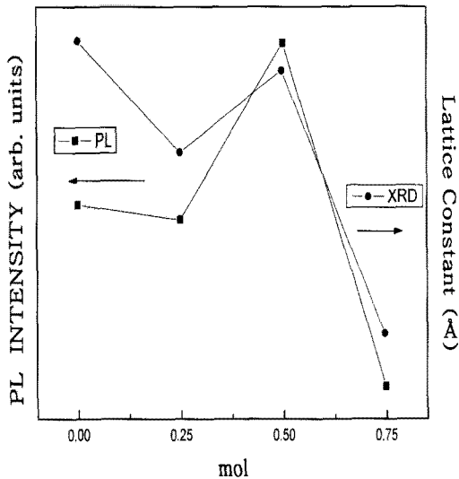
그림 6. x의 변화에 따른 (Zn_{1-x}Mg_x)_2SiO_4:Mn PL 발광 세기와 격자상수와의 관계.
