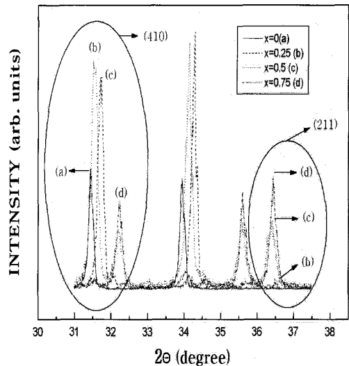
그림 3. x의 변화에 따른 (Zn 1-x Mg x ) 2 SiO 4 :Mn (410)면과 (211)면의 XRD 패턴.
