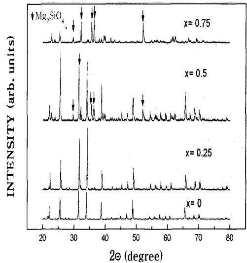
그림 2. Mg 농도에 따른 (Zn 1-x Mg x ) 2 SiO 4 :Mn 형광체의 XRD.
