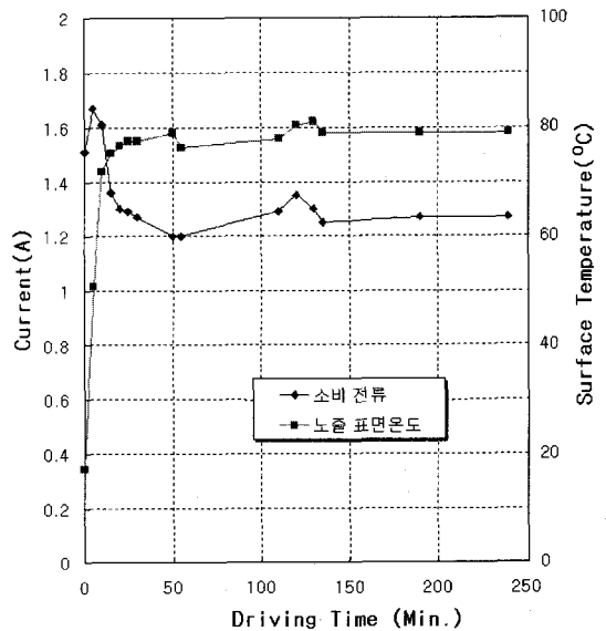
그림 4. 초음파 노즐의 소비전류 및 표면온도.
