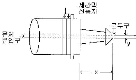
그림 1. 초음파 노즐의 형상.
