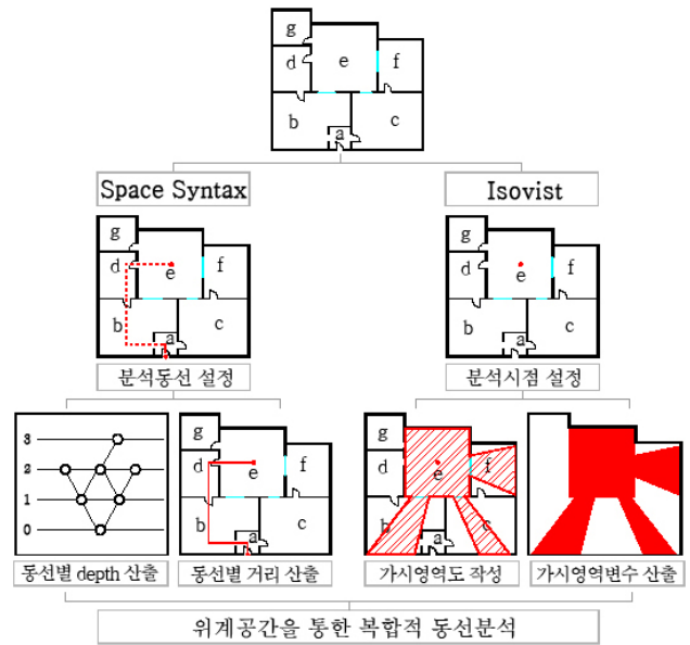
그림1. 분석 프로세스
