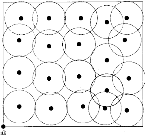
그림 4. VFA를 이용했을 때 각 센서의 감지 담당 범위
