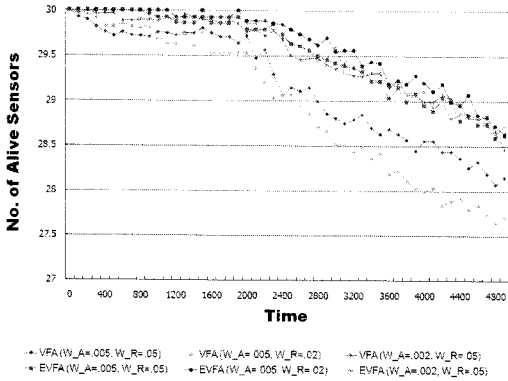
그림 10. 동작 중인 센서 수의 변화 추이
