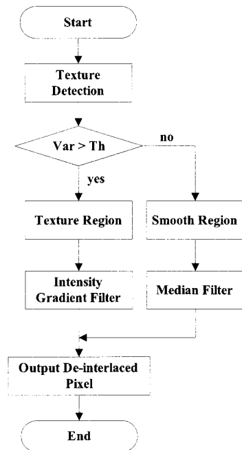
그림 3. 제안하는 알고리즘의 흐름도.
