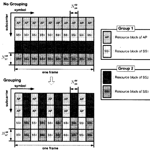
그림 5. 그룹핑 적용 유무에 따른 SDD 방식의 프레임 구조의 예 자원블록에 포함되는 심볼에 삽입하고, 자원블록 양 끝 심볼의 CS 길이는 인접 그룹에 속한 AP 혹은 SS를 포함하여 새로운 그룹을 생성한 후에 새로운 그룹의 최대 상호 시간 지연과 최대 채널 지연 길이를 고려하여 설정한다. 이를 수학식으로 나타내면 다음과 같다.
