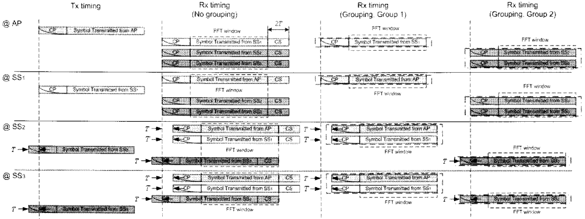
그림 2. 그룹핑 적용 유무에 따른 AP와 각 SS의 송신 시간과 수신 시간
