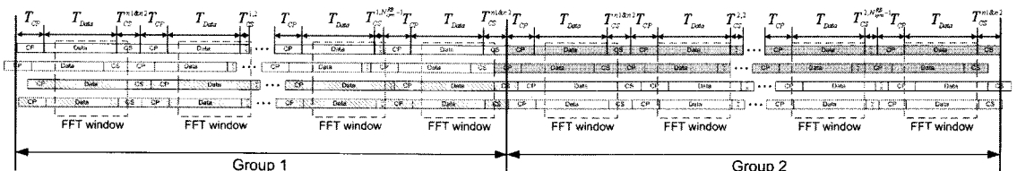
그림 6. 두 그룹 사이의 자원 블록의 양 끝 심볼 구조
