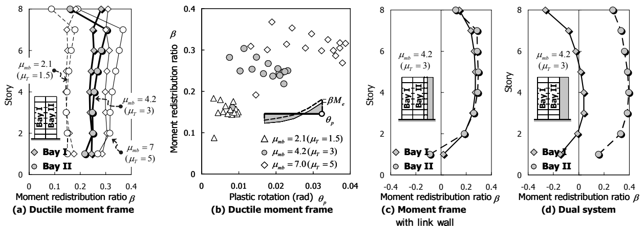
〈그림 9〉 설계연성도와 모멘트재분배율의 관계
