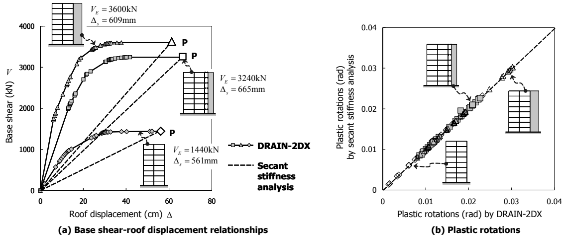
〈그림 10〉 할선강성해석을 이용한 내진설계 결과 검증
