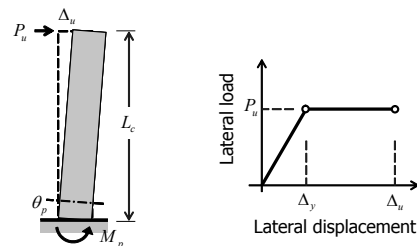
〈그림 3〉 켄틸레버 부재의 변형
