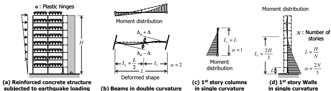
〈그림 4〉 소성변형의 분포 및 거동특성에 따른 부재활선강성의 결정
