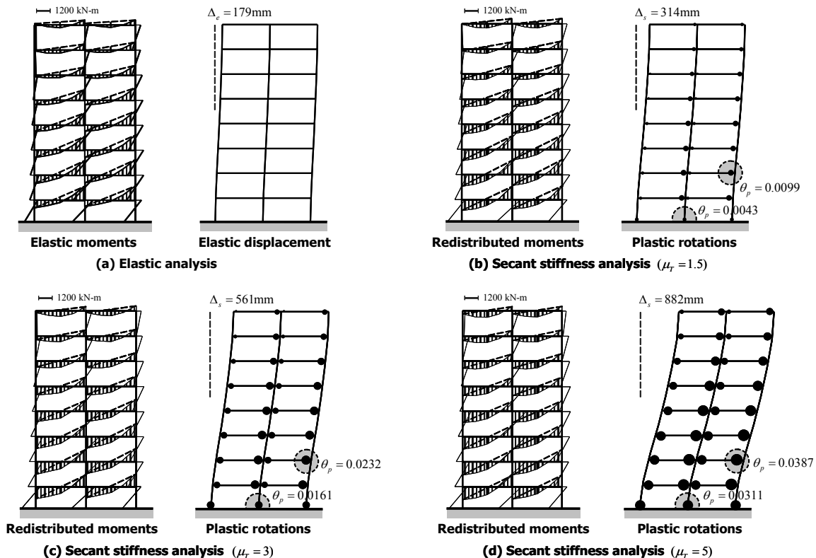
〈그림 6〉 할선강성해석을 이용한 모멘트골조의 내진설계
