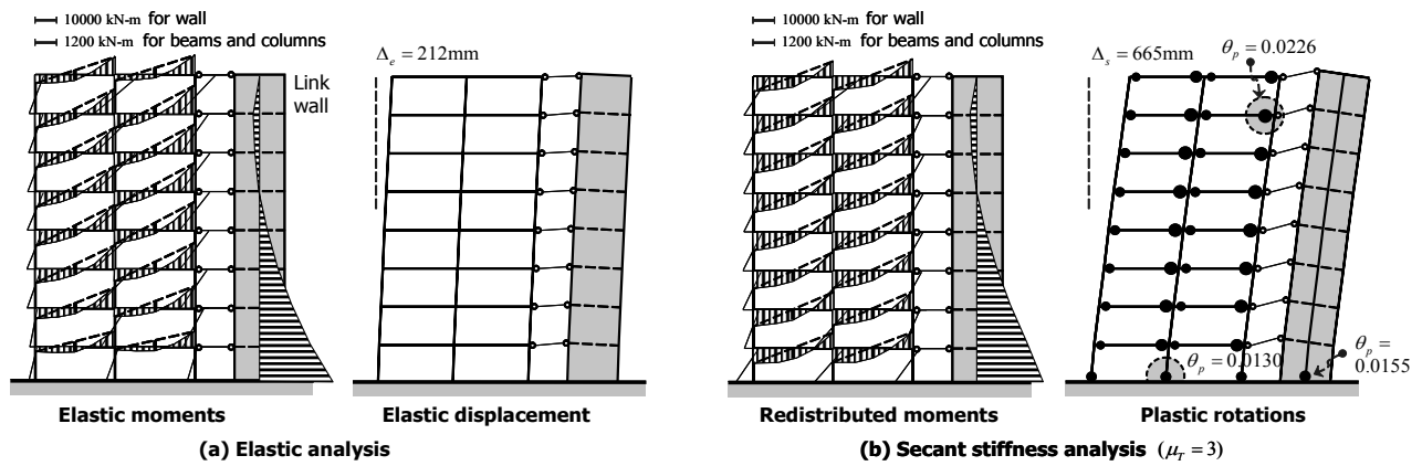
〈그림 7〉 활선강성해석을 이용한 모멘트골조와 전단벽이 링크보로 연결된 이중골조의 내진설계
