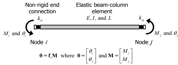
〈그림 2〉 비강접 단부접합부를 갖는 보-기둥요소(NREC요소)
