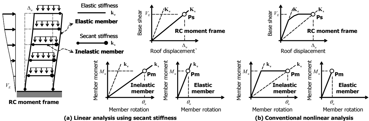
〈그림 1〉 할선강성해석을 이용한 설계개념
