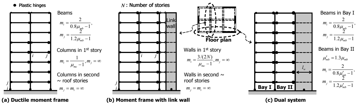
〈그림 5〉 구조해석을 위한 연성골조 및 이중골조의 활선강성모델
