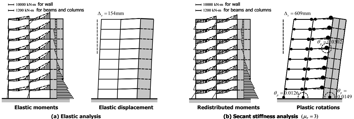
〈그림 8〉 활선강성해석을 이용한 이중골조의 내진설계
