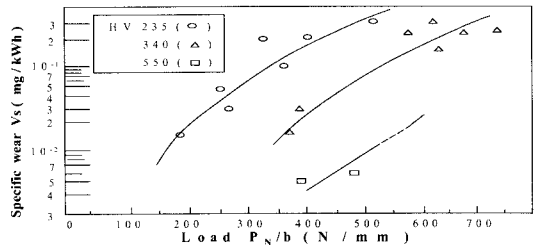
[그림 9] 경도에 따른 하중과 비마모량의 영향
