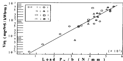
[그림 5] 하중과 점성계수 및 비마모량의 영향
