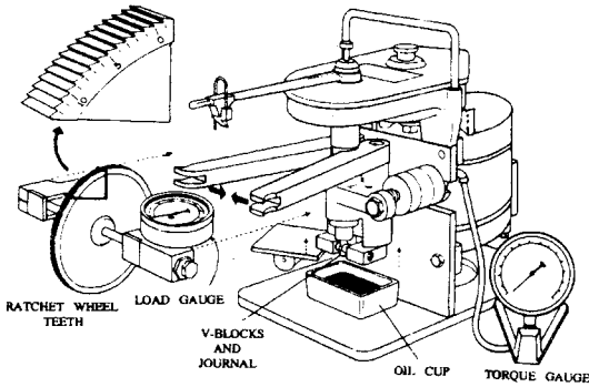
[그림 1] 마찰 마모 실험장치
