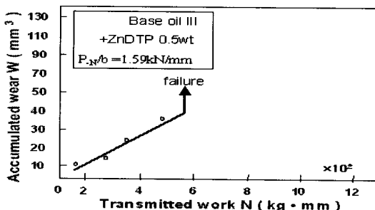
[그림 3] 비마모량 곡선
