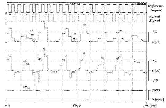
(a) 가감속이 없는 경우(5,000[rpm])
