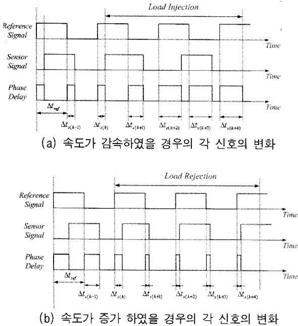
그림 4 속도 변동에 대한 각 신호의 변화 Fig. 4 Waveforms of reference, hall-sensor and phase delays according speed variation
