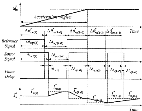
그림 5 제안된 방식에서의 지령속도 변동 Fig. 5 Current variation of the proposed control method
