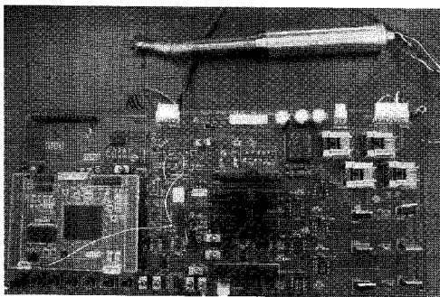
그림 7 실험 환경 Fig. 7 Experimental configuration
