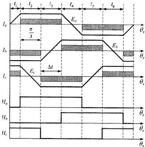
그림 2 BLDCM의 역기전력, 입력전류 및 홀센서 신호 Fig. 2 Waveforms of back e.m.f, input current and hall sensor signals of BLDCM
