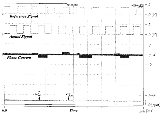
그림 8 2,000[rpm]에서의 실험결과 Fig. 8 Experimental result at 2,000[rpm]
