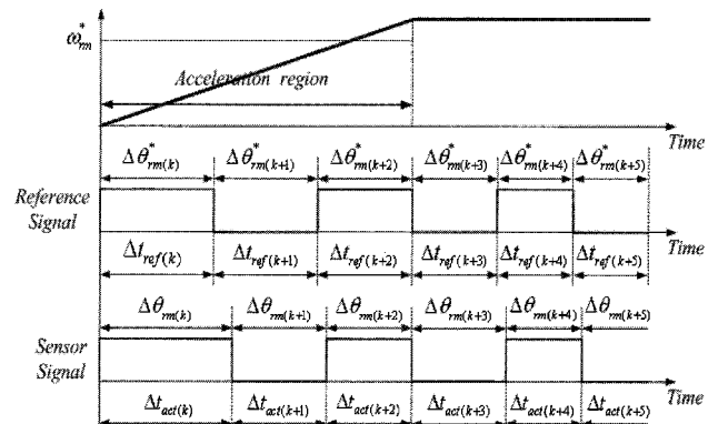
그림 3 속도 지령에 따른 지령 신호와 실제 홀센서 신호 Fig. 3 The reference pulse according to speed reference and actual hall sensor signal
