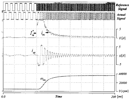
그림 11 속도 지령 변동에 대한 실험결과 (5,000[rpm] → 38,000[rpm]) Fig. 11 Experimental result according to speed variation(5,000[rpm] → 38,000[rpm])
