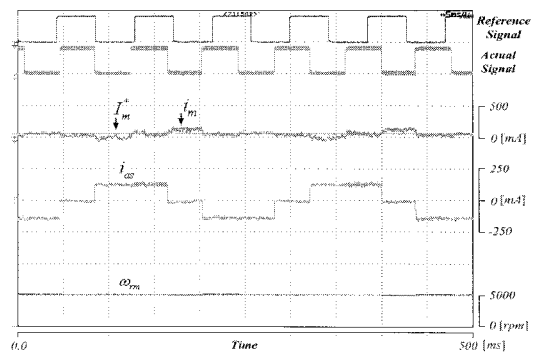
그림 9 정상상태 실험결과(5,000[rpm] 무부하) Fig. 9 Experimental result in steady state (5,000[rpm] no-load)
