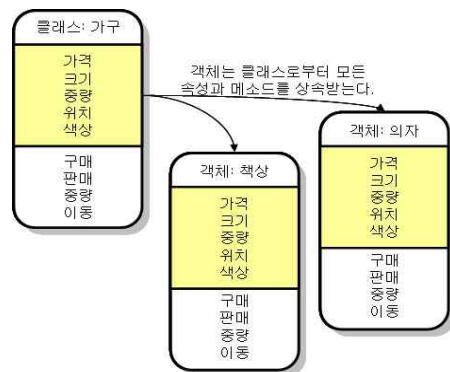
(그림 2) 상속성의 개념
