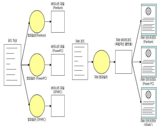
(그림 4) 고전적인 컴파일(좌)과 자바 컴파일(우)
