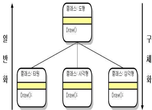
(그림 3) 메소드의 다형성
