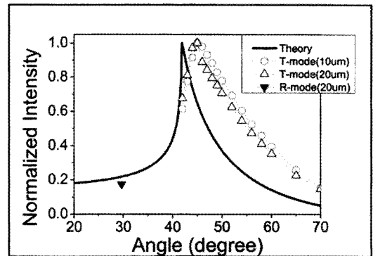
그림 5. 공기와 프리즘 계면에서 형성되는 각도별 전기장 세기에 대한 이론적인 그래프(실선)와 이에 해당하는 각도에서 계산한 최대 산란광 세기 비교 그래프(심볼).
