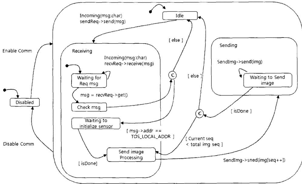
그림 3. 이미지 전송 상태 다이어그램. Fig 3. State diagram of image transmit
