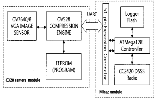
그림 2. 이미지 센서와 통신 모트 간 구성도. Fig 2. Configuration between image sensor and mote
