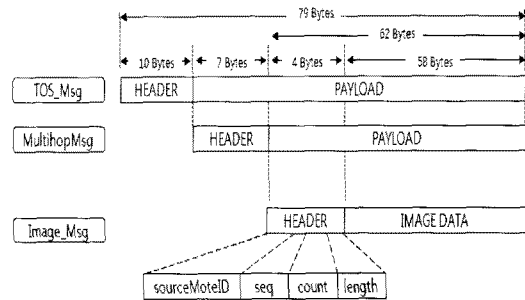
그림 5. 이미지 전송 메시지. Fig 5. Image transmit message
