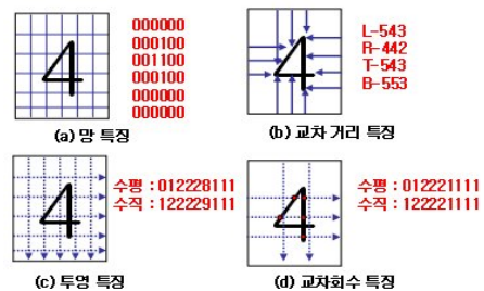
(그림 13) 격자 및 거리 특징 추출
