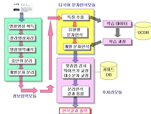
(그림 1) 다국어 명함인식기의 구성도
