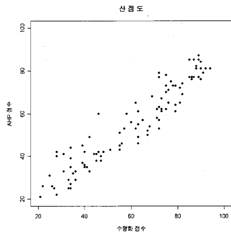
<그림 5> 수량화 점수와 AHP점수 산점도
