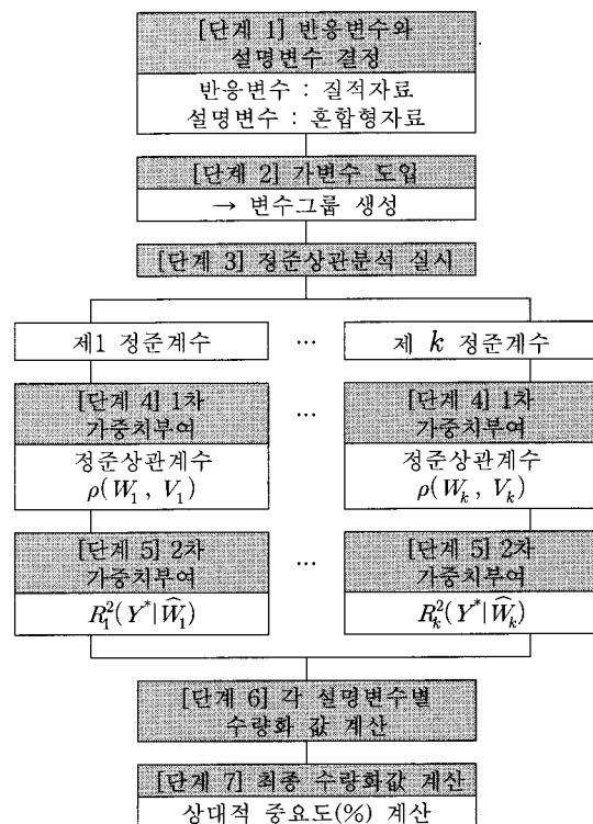
<그림 1> 수량화II 분석 과정
