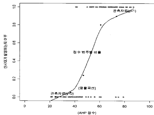
<그림 4> AHP 점수와 산사태 발생비율
