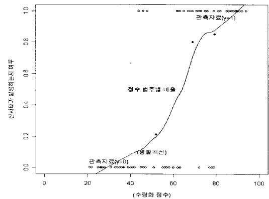
<그림 3> 수량화 점수와 산사태 발생비율
