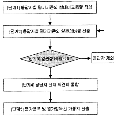
<그림 2> AHP 분석 절차
