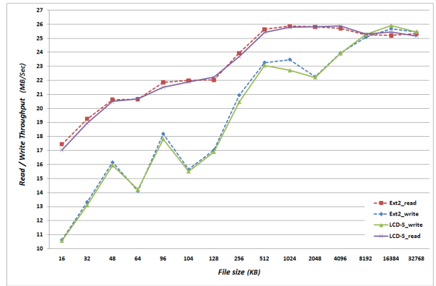
(그림 10) File Operation1에서의 읽기/쓰기 성능 비교
