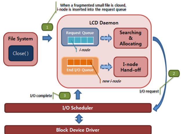
(그림 6) LCD-FS 설계
