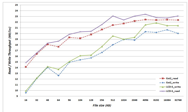
(그림 11) File Operation10에서의 읽기/쓰기 성능 비교
