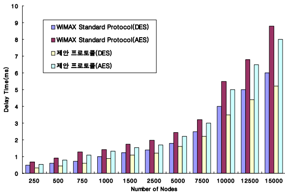
(그림 5) 노드 수 증가와 암호 알고리즘에 따른 인증 지연시간
