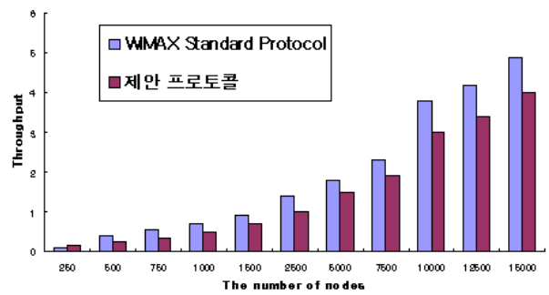
(그림 7) 노드 수에 따른 인증 서버의 처리량
