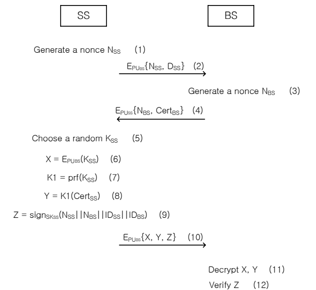
(그림 2) 가입자와 베이스 스테이션 사이의 초기 인증 프로토콜
