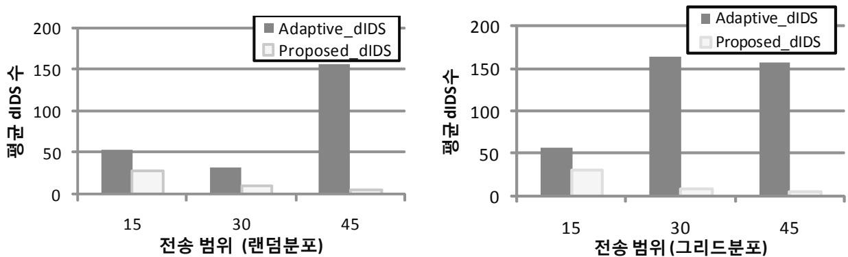
(그림 8) 전송범위에 따른 평균 dIDS 수
