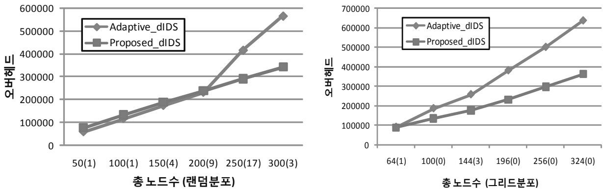
(그림 9) 총 노드수에 따른 오버헤드
