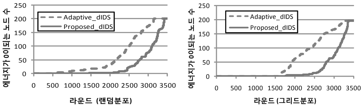
(그림 7) 각 라운드의 에너지가 0이 되는 노드 수
