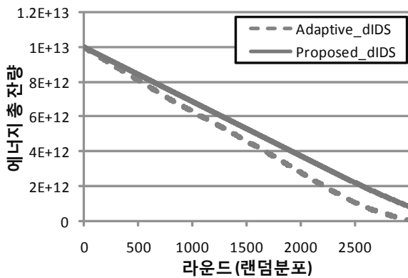
(그림 5) 각 라운드의 에너지 총 잔량
