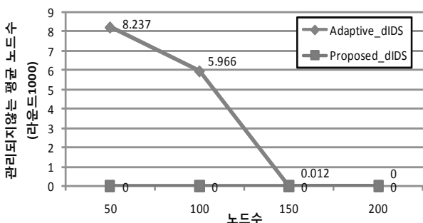
(그림 11) 총 노드수당 관리되지 않는 평균 노드 수
