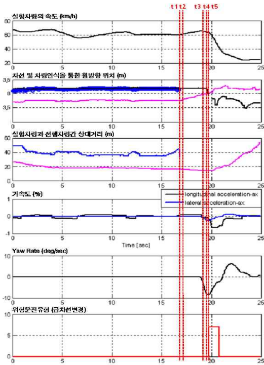
<그림 13> 급차선 변경 실험 결과 <Fig. 13> Vehicle behavior under sudden lane change
