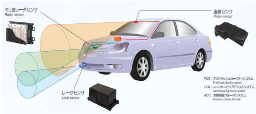
<그림 3> Denso 센싱 시스템 구성도 <Fig. 3> Configuration of Denso sensing system
