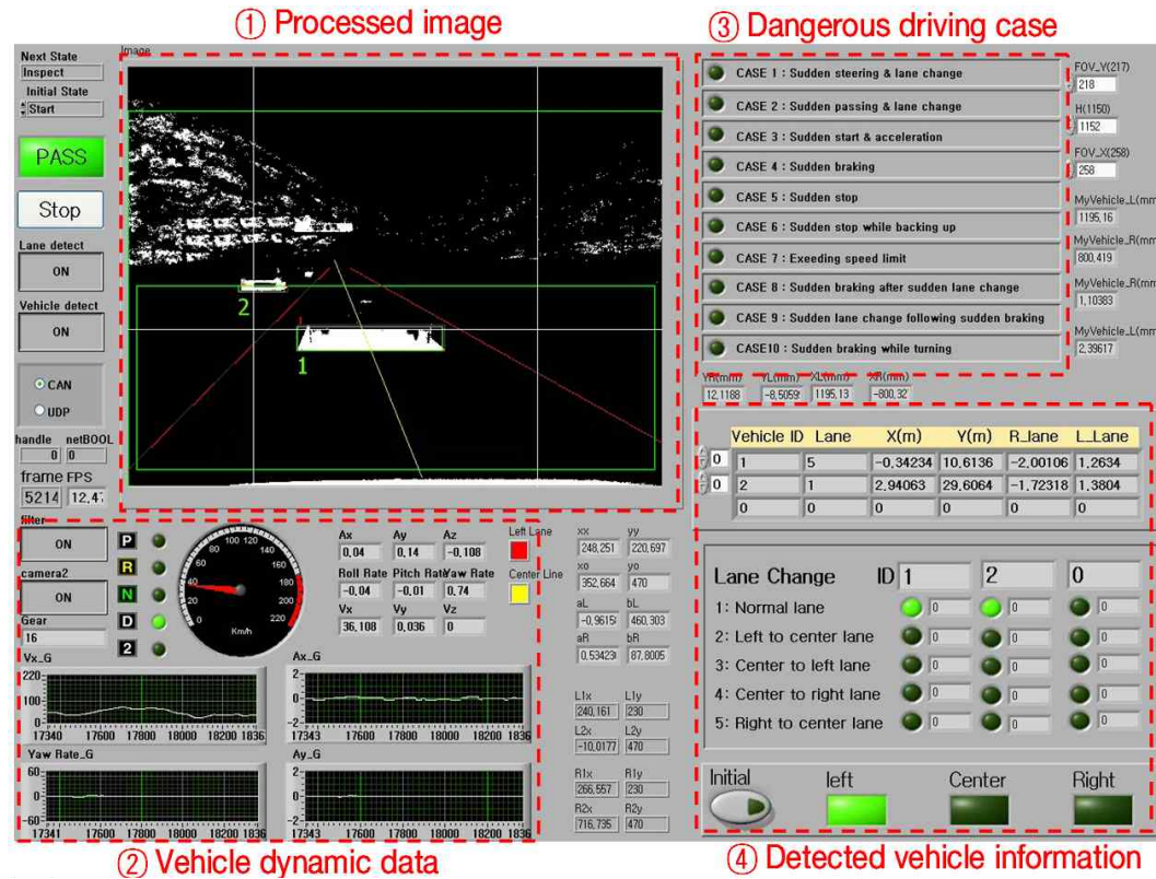
<그림 8> Vision 시스템 메인 프로그램 GUI <Fig 8> Vision system main program GUI
