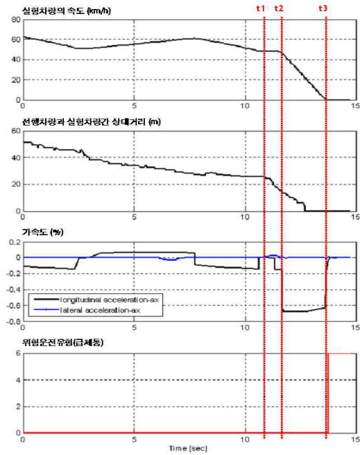
<그림 11> 급정지 실험 결과 <Fig. 11> Vehicle behavior under sudden stop
