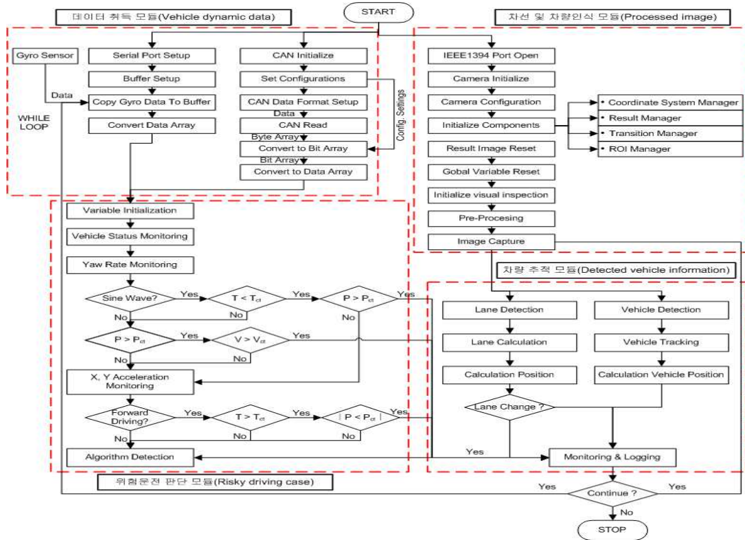
<그림 4> Vision 시스템 알고리즘 <Fig. 4> Algorithm of Vision system
